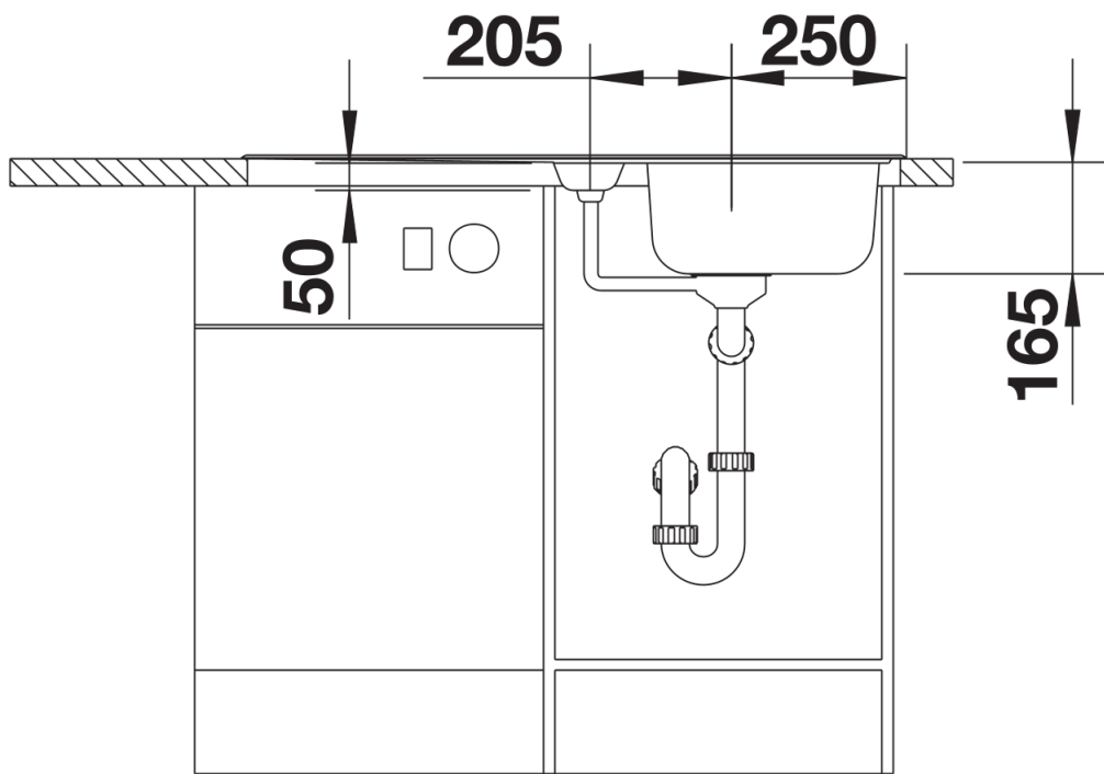
Frontansicht
