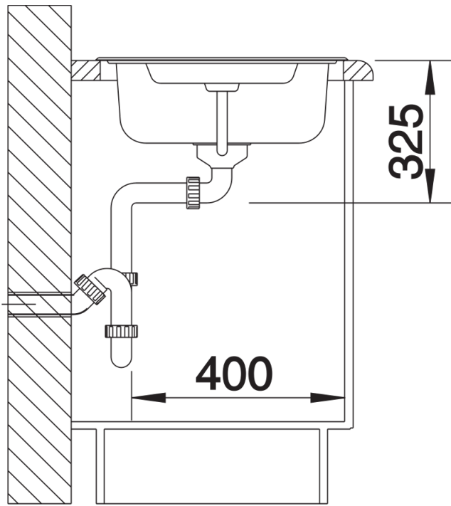
Seitenansicht
