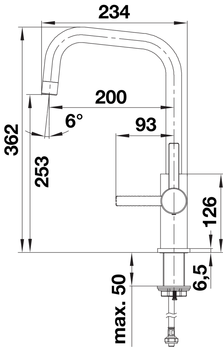
Seitenansicht
