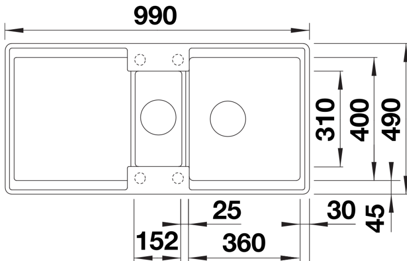
Aufsicht
