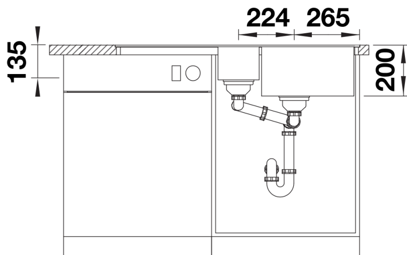
Frontansicht
