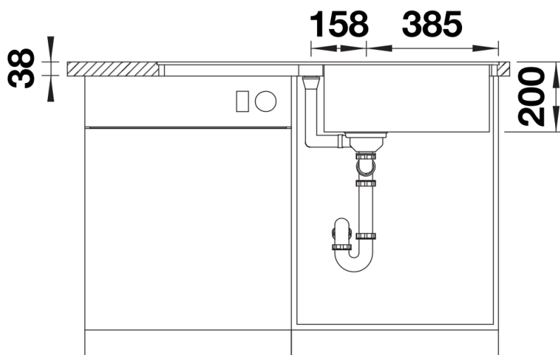
Frontansicht
