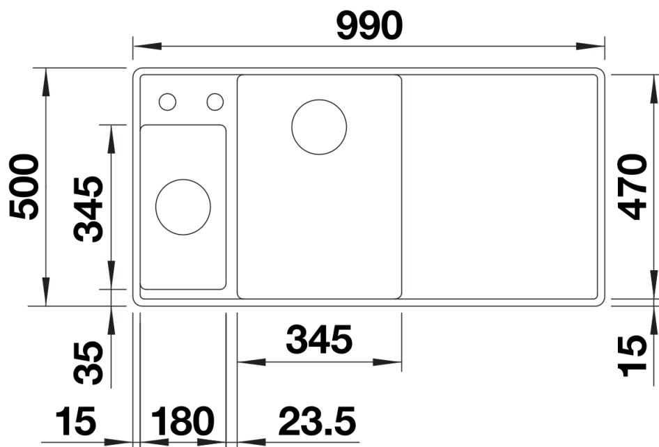
Aufsicht
