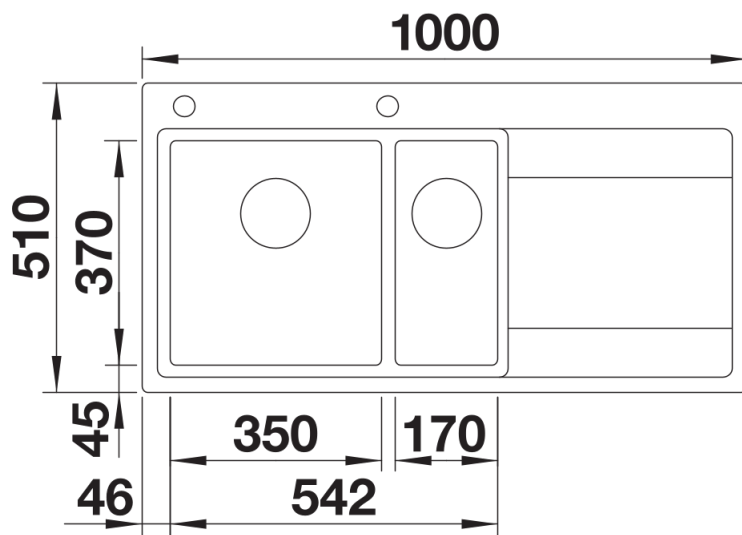
Aufsicht
