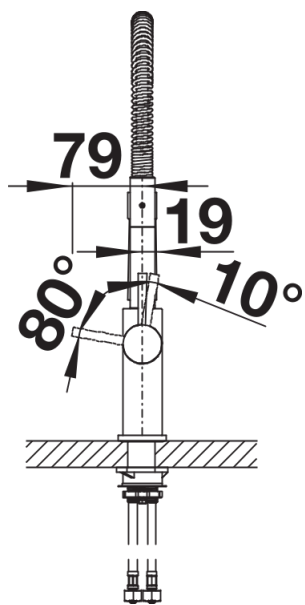
Seitenansicht Hebel 2D
