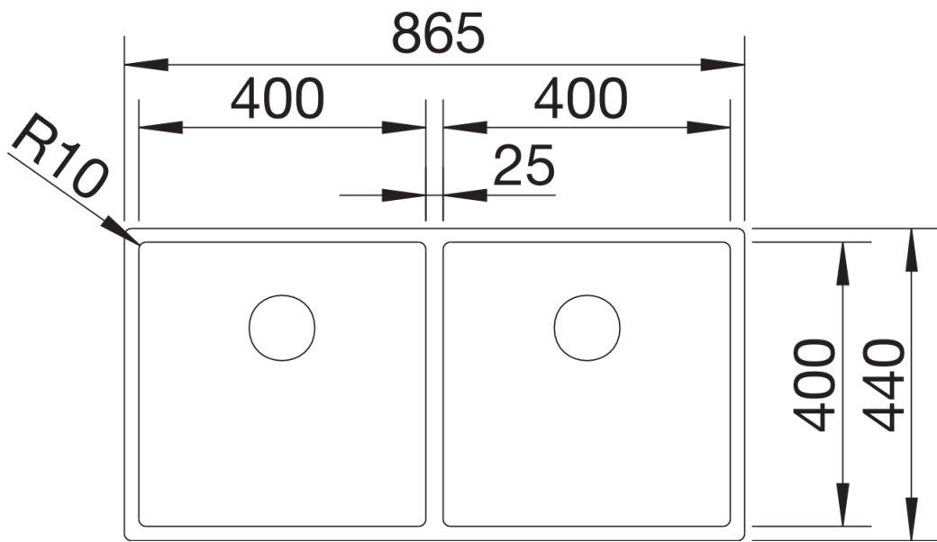
Aufsicht
