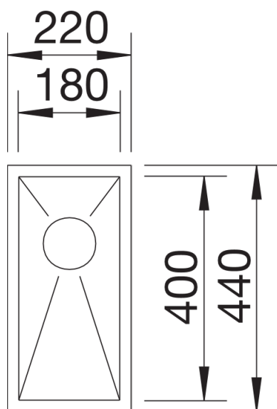
Aufsicht
