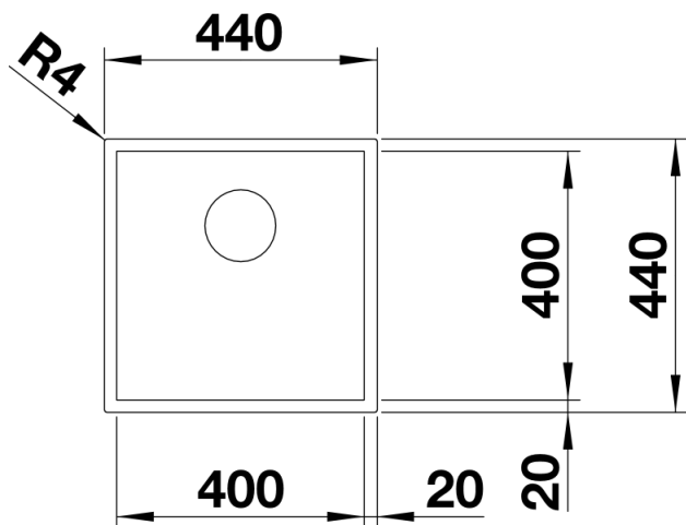
Aufsicht
