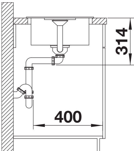
Seitenansicht
