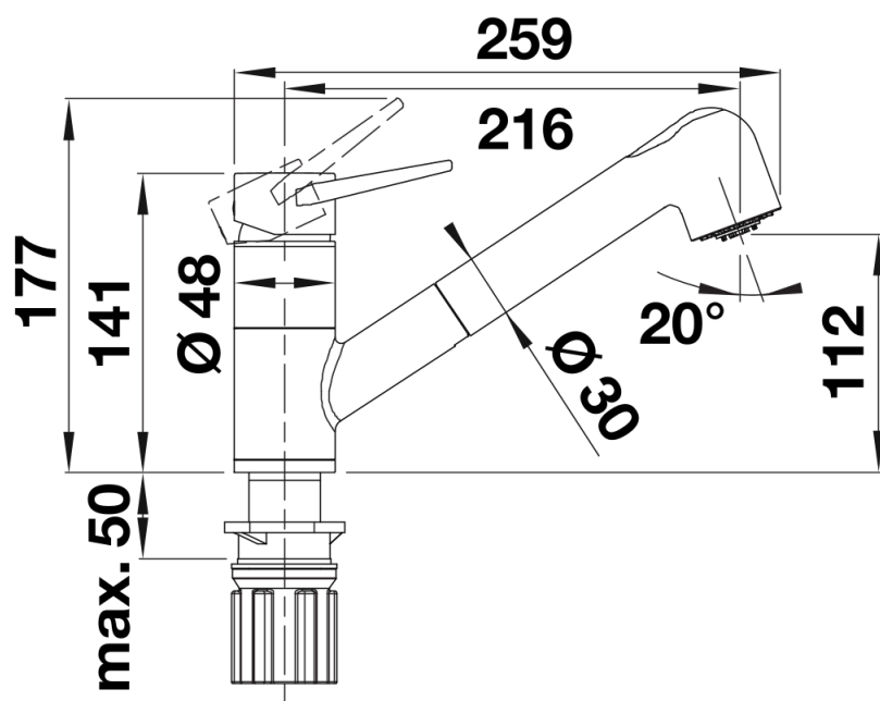
Vue latérale
