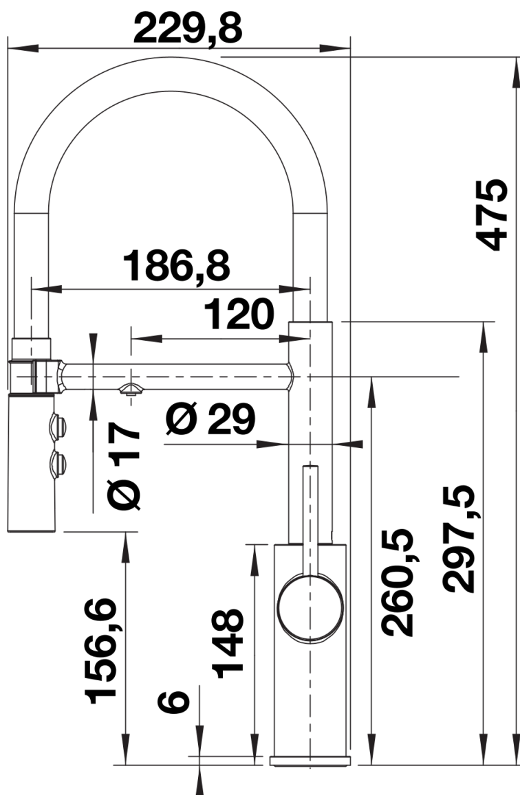
Vue latérale
