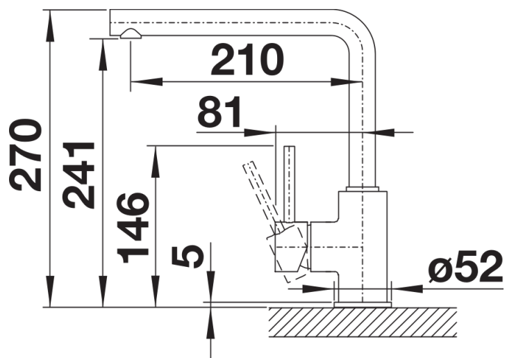
Vue latérale
