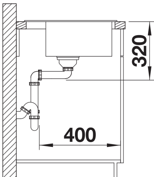
Vue latérale
