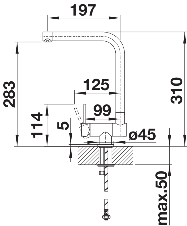
Vue latérale
