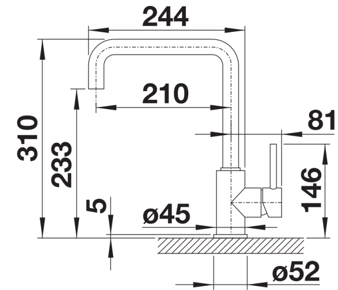
Vue latérale
