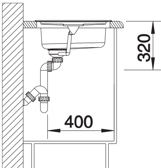
Vue latérale
