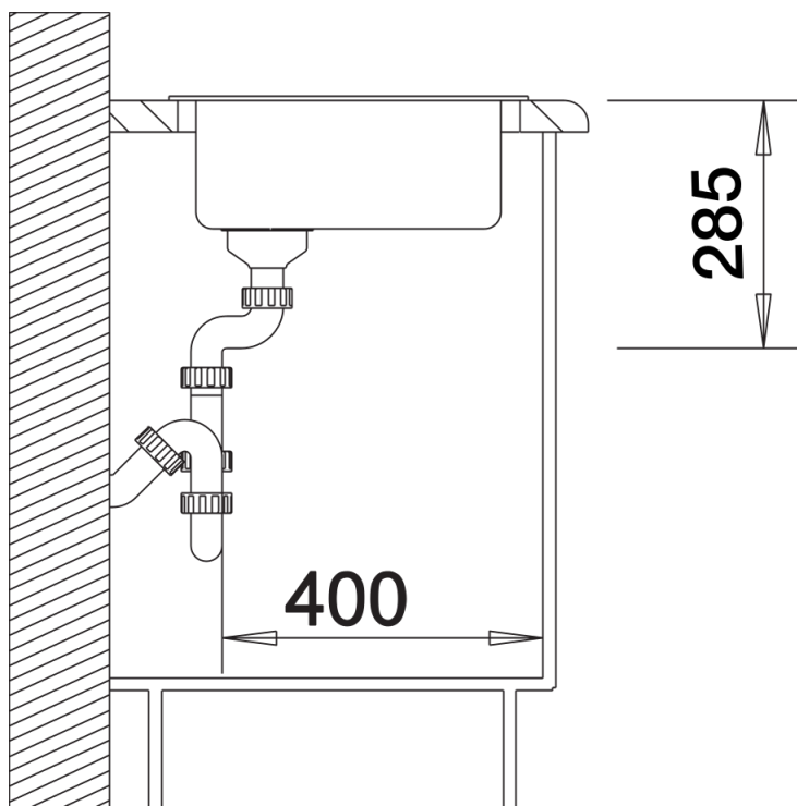
Vue latérale
