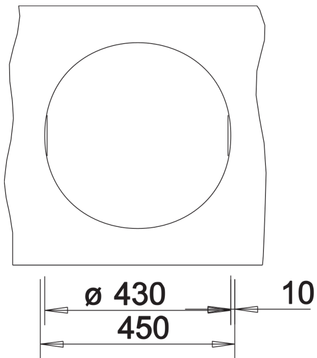
Découpe
