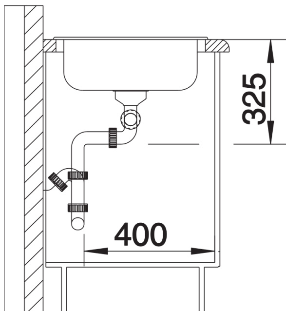
Vue latérale
