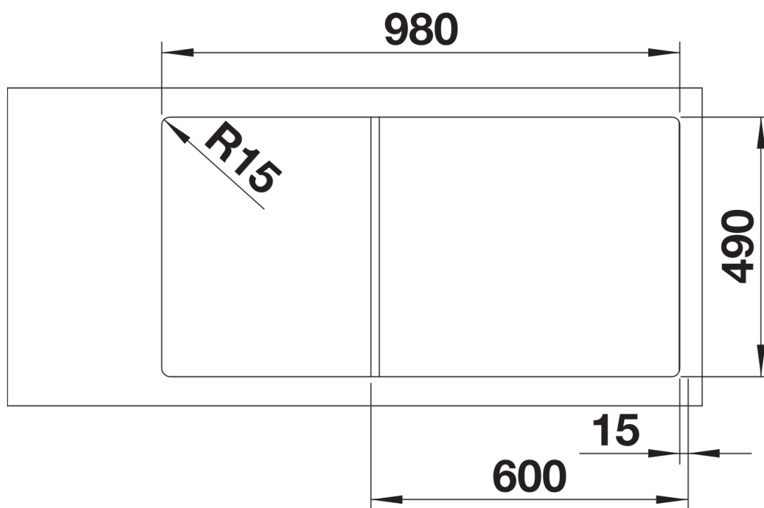
Découpe
