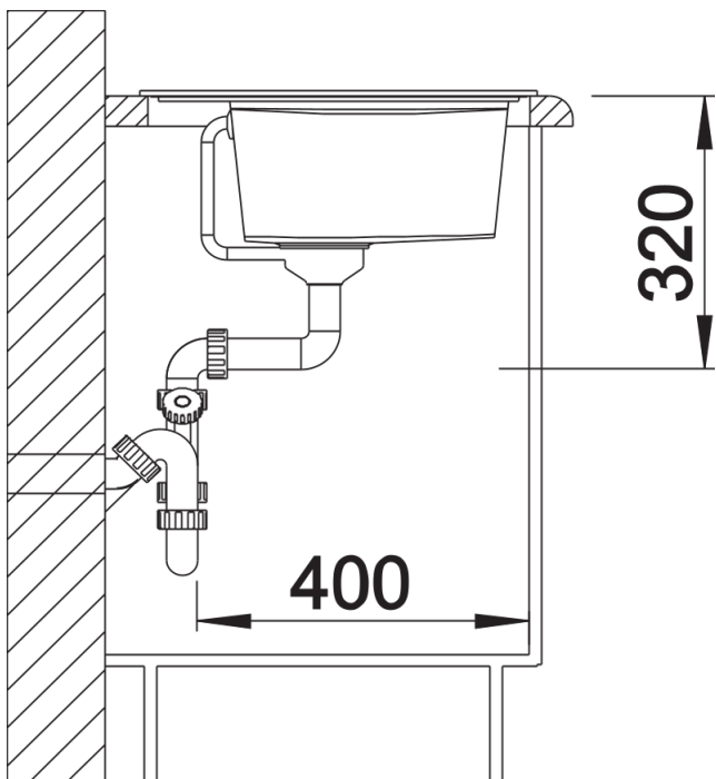
Vue latérale
