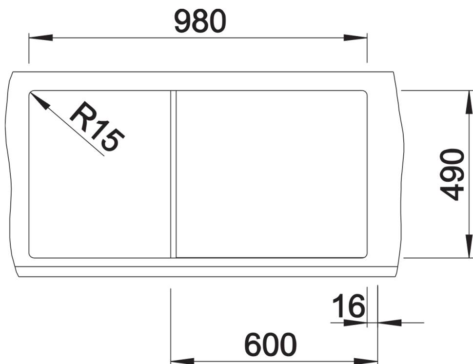
Découpe
