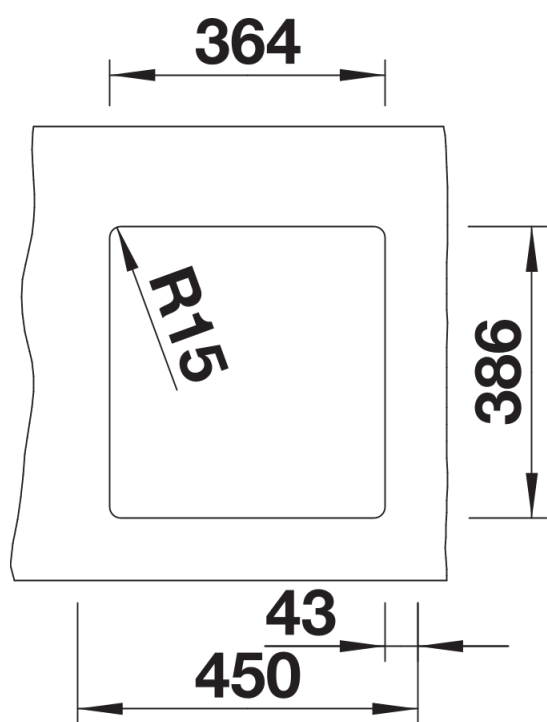
Découpe
