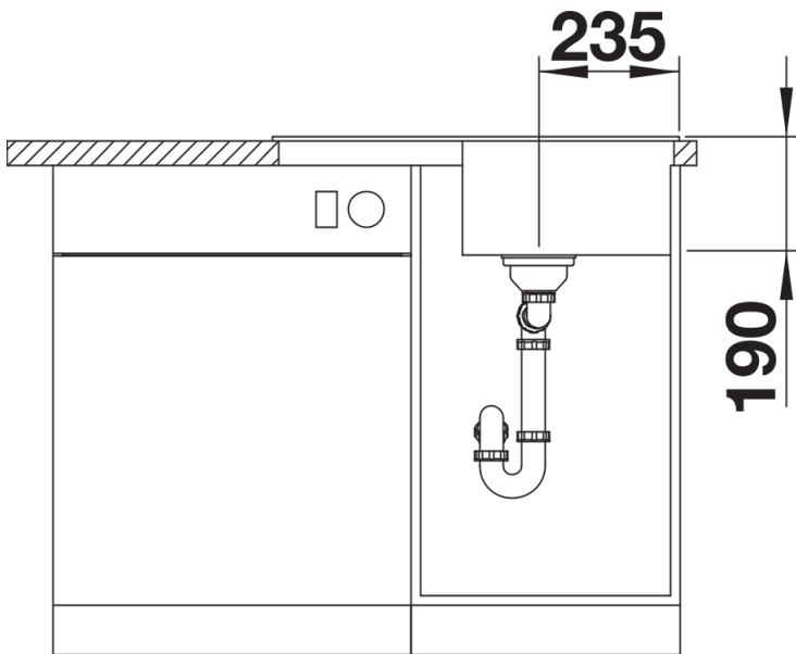
Vooraanzicht
