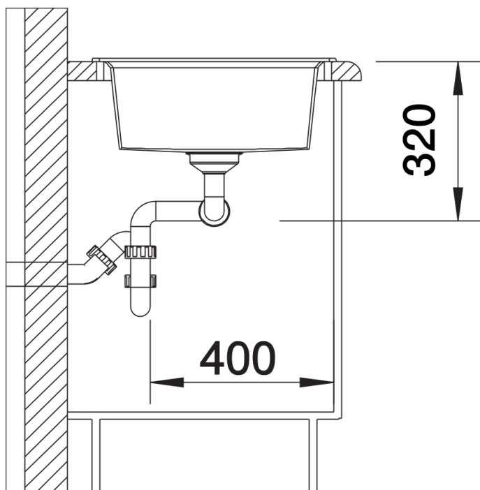
Zijaanzicht
