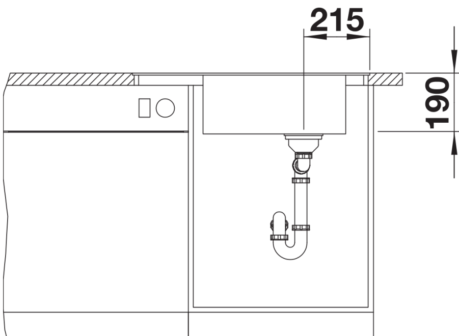
Vooraanzicht
