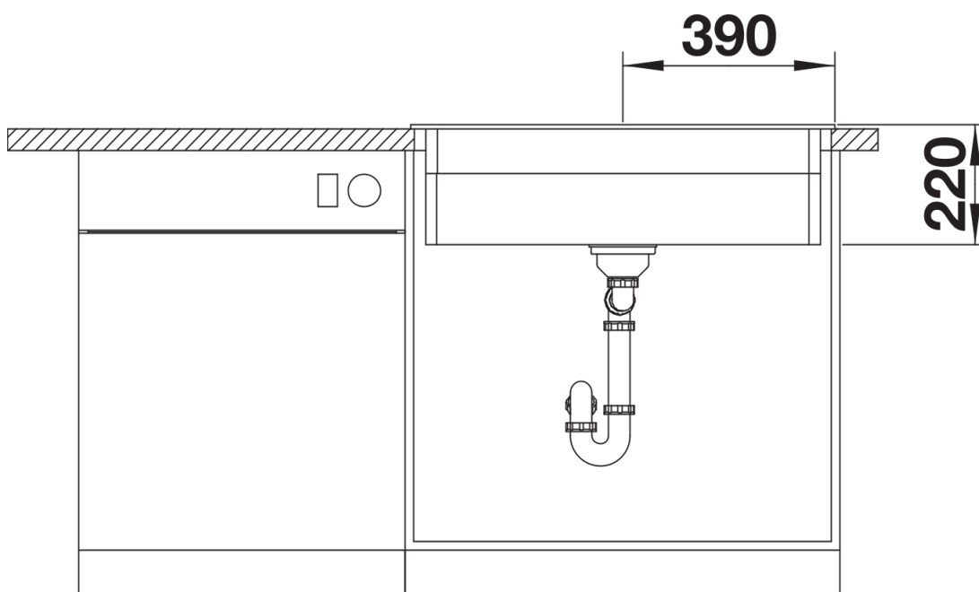
Vooraanzicht
