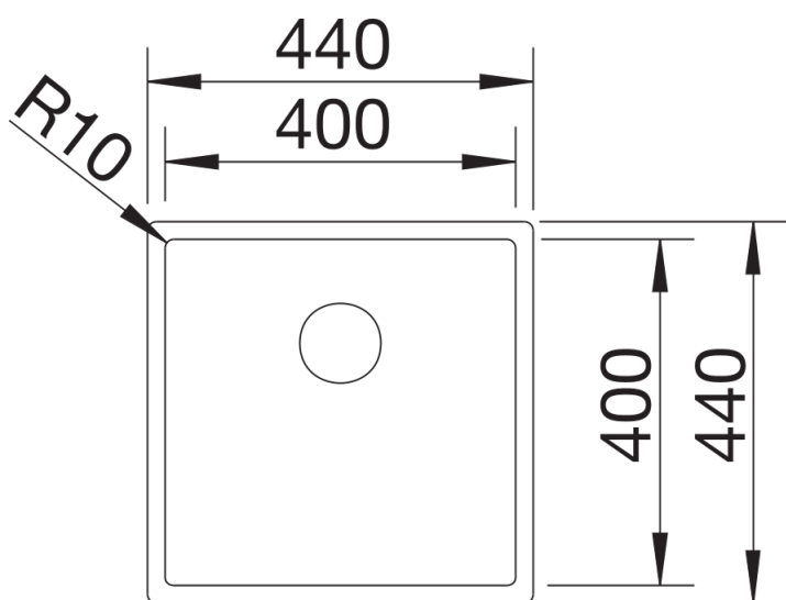
Bovenaanzicht
