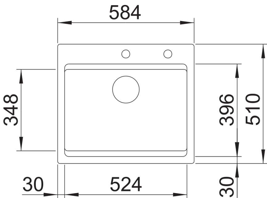
Bovenaanzicht
