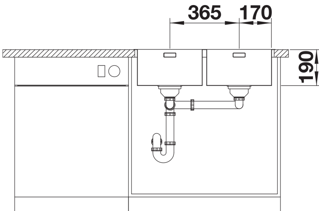
Vooraanzicht
