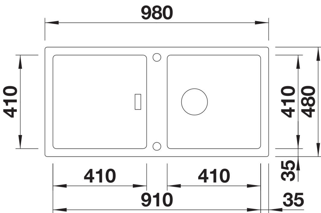
Bovenaanzicht
