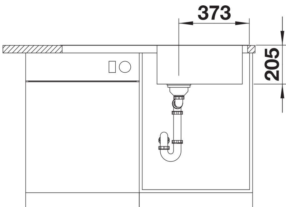
Vooraanzicht
