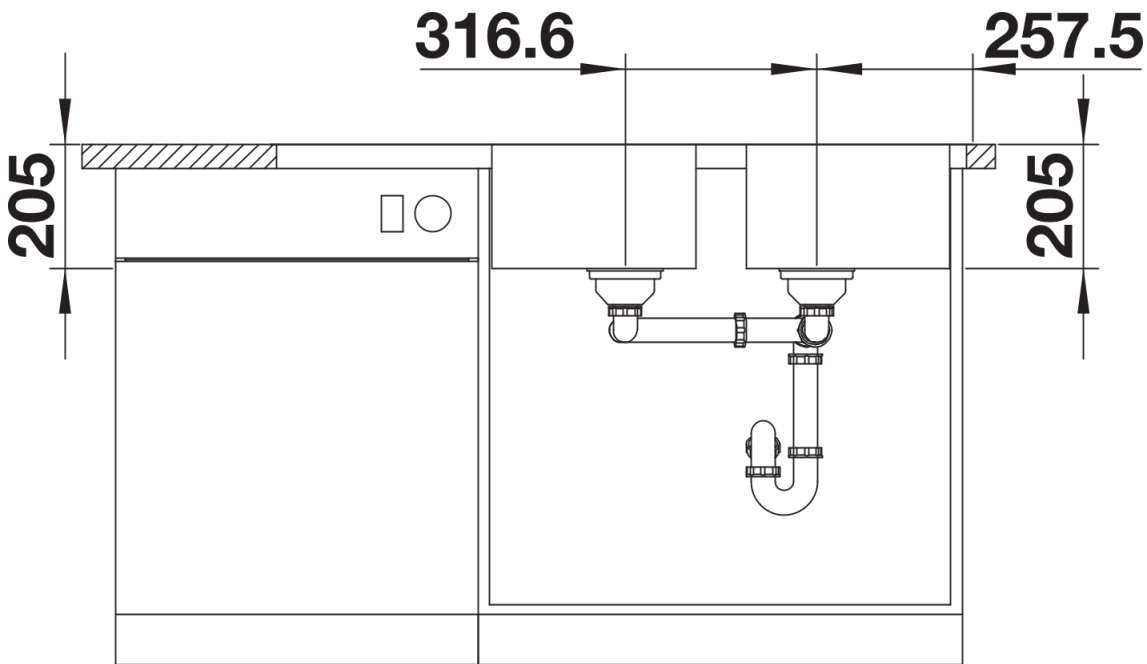
Voorraanzicht
