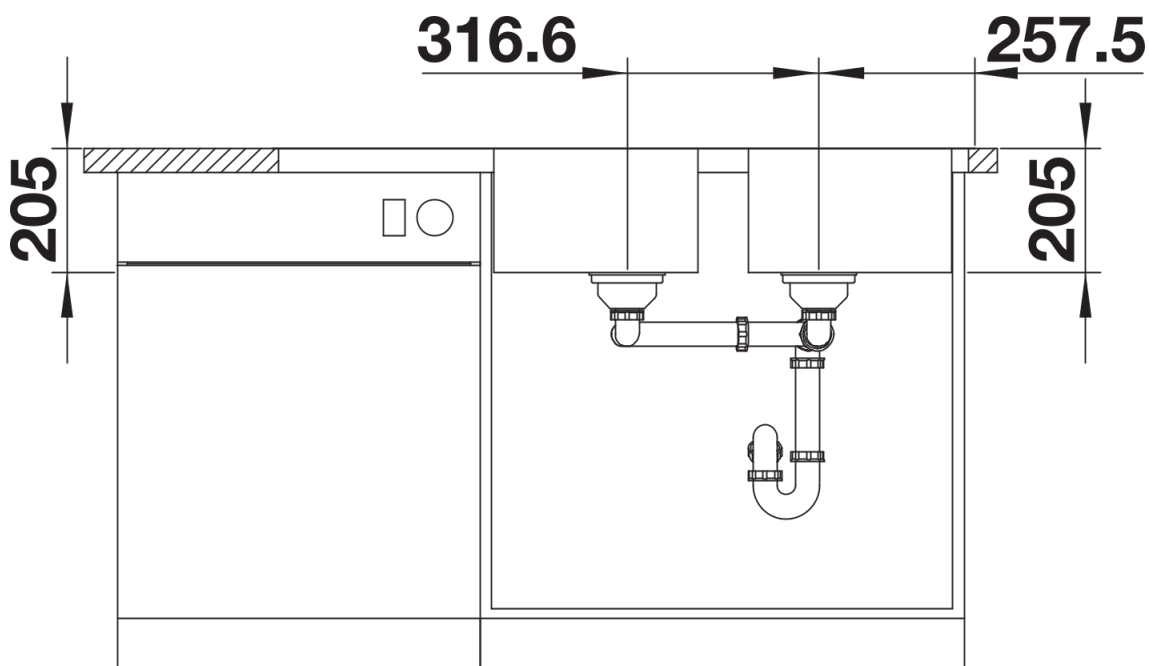
Vooraanzicht
