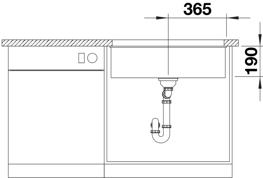
Vooranzicht
