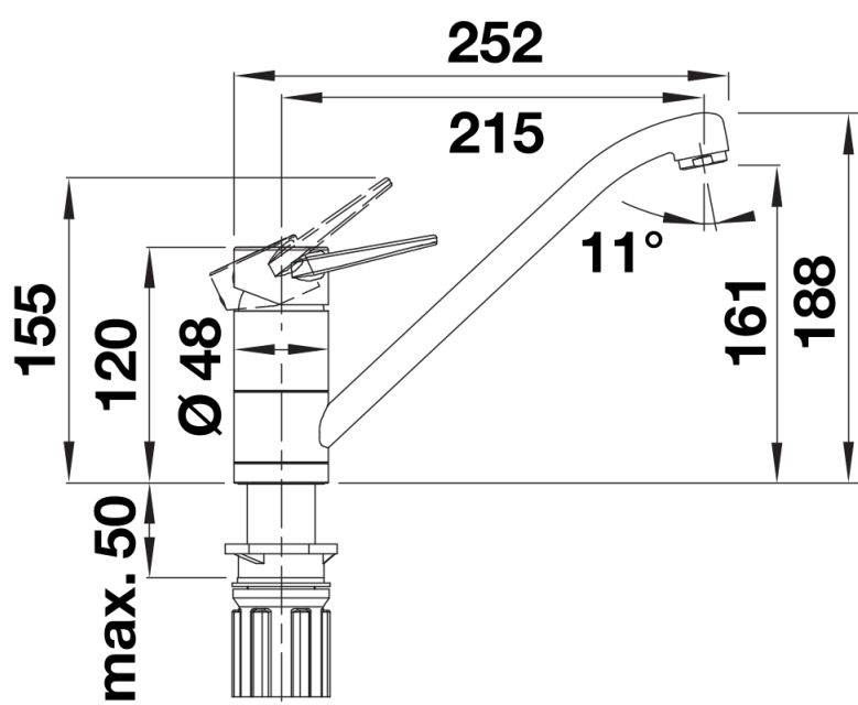
Zijaanzicht
