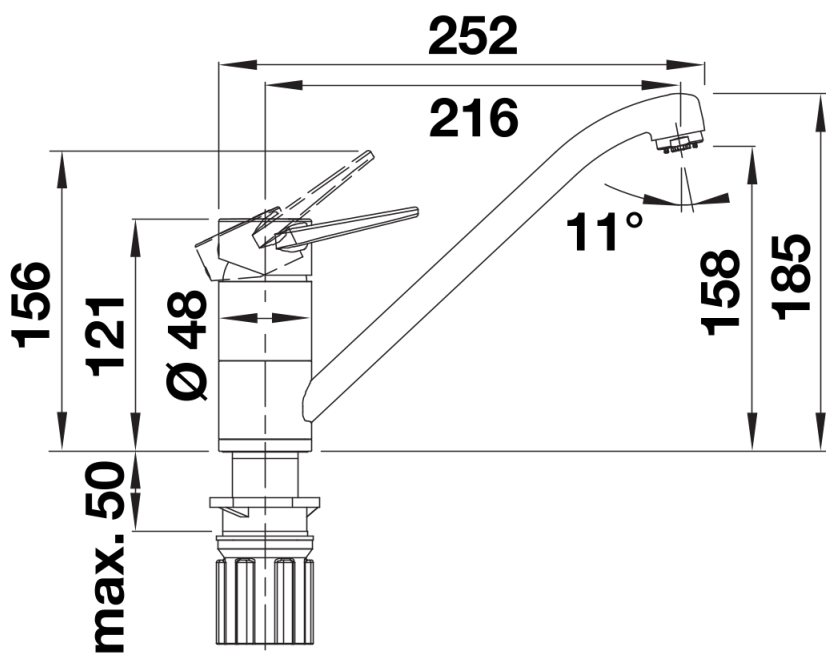
Zijaanzicht
