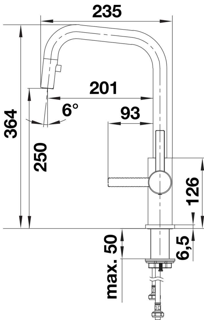
Zijaanzicht
