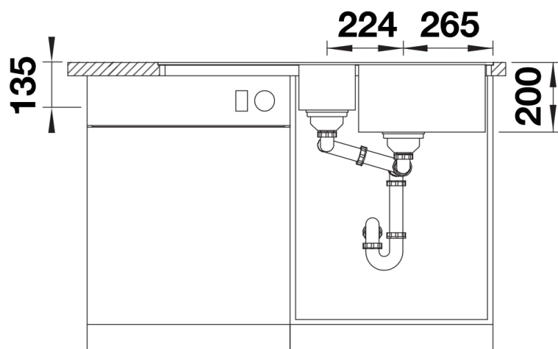
Vooraanzicht
