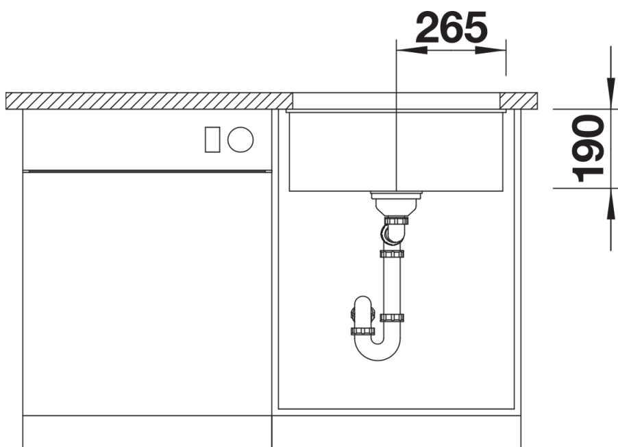
Vooraanzicht
