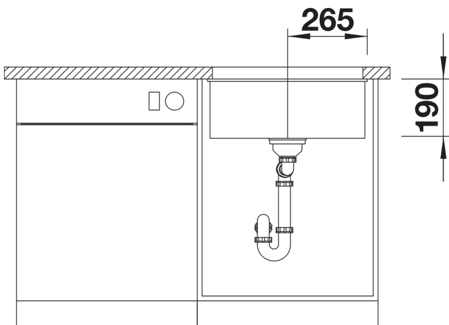
Vooraanzicht
