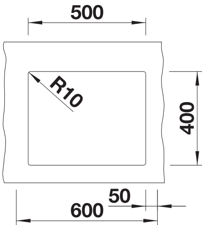
Uitgesneden
