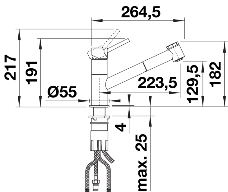
Zijaanzicht
