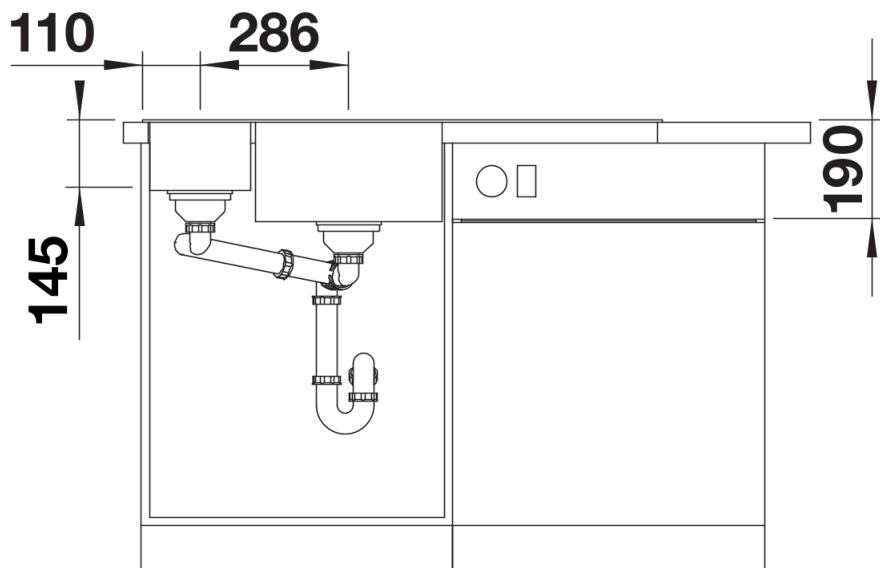
Vooraanzicht
