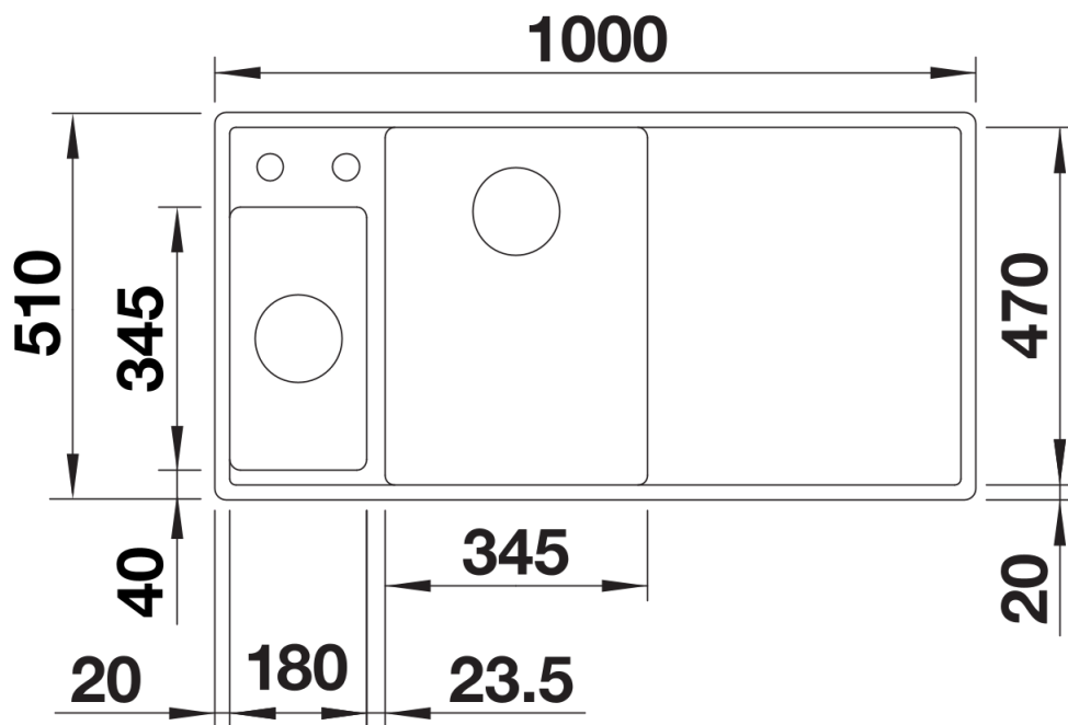
Bovenaanzicht
