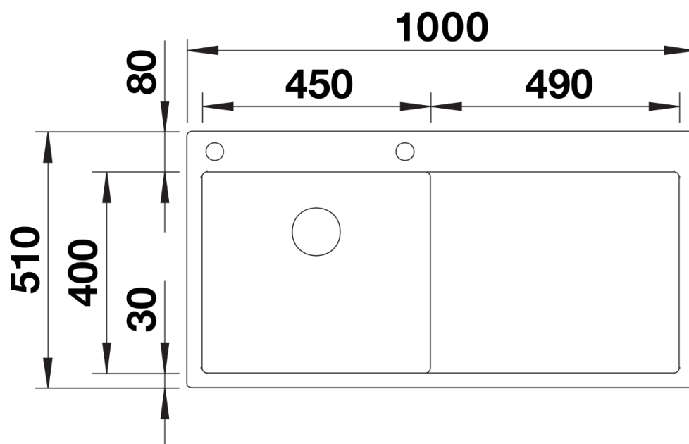
Bovenaanzicht
