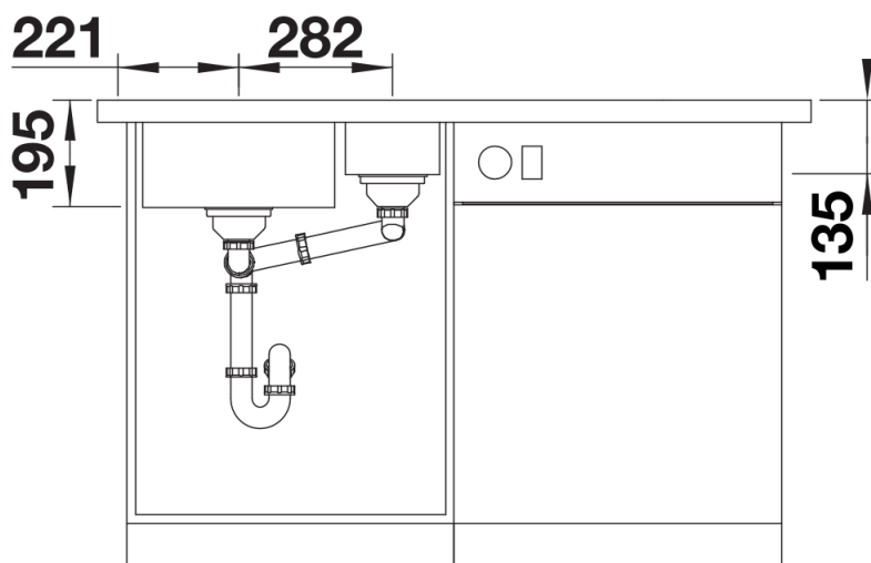
Vooraanzicht
