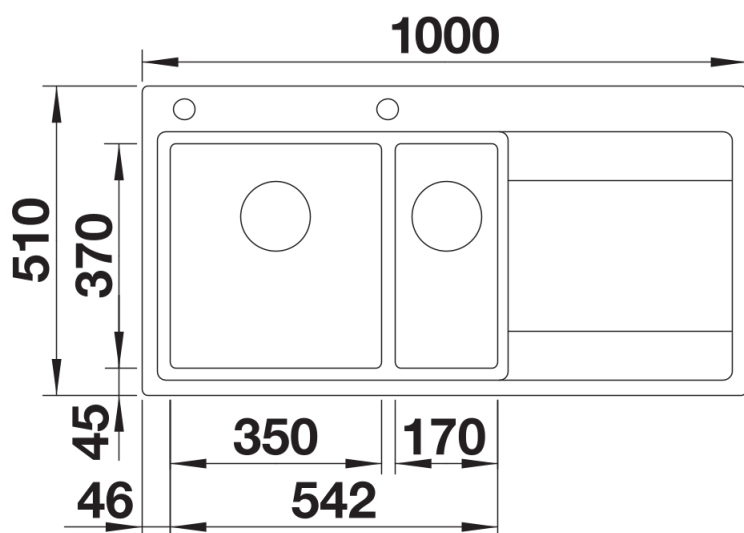
Bovenaanzicht
