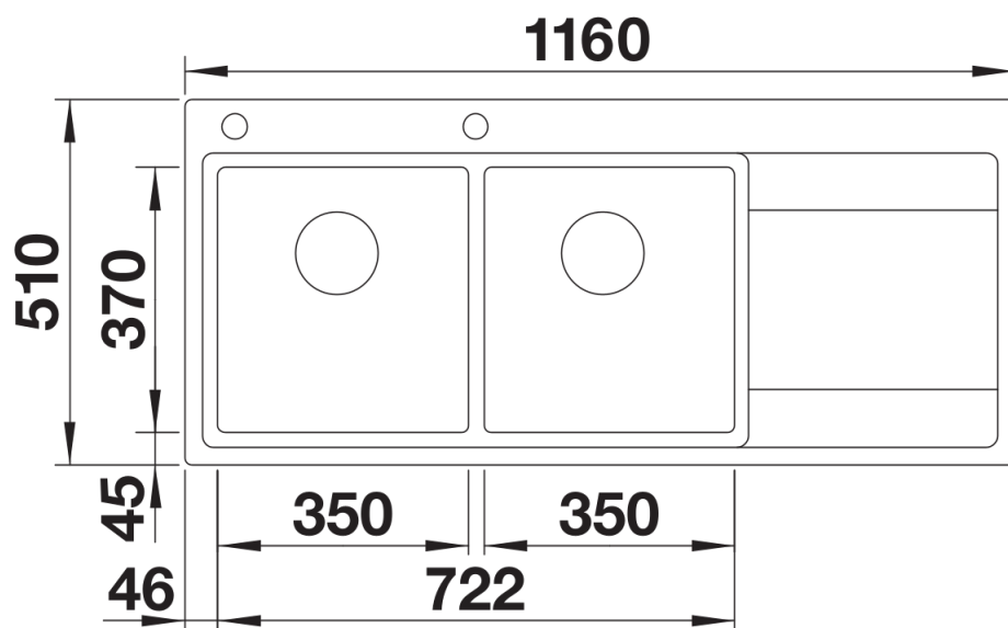
Bovenaanzicht
