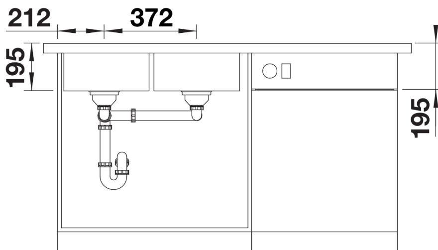
Vooraanzicht
