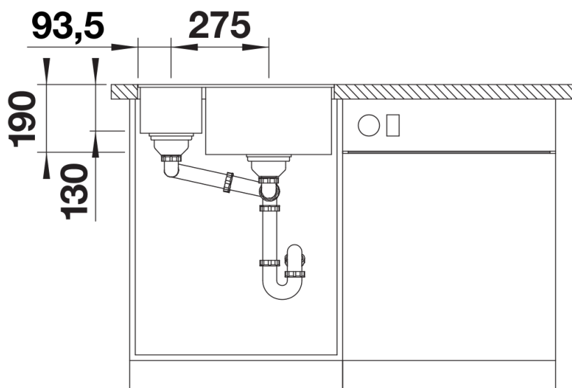
Vooraanzicht
