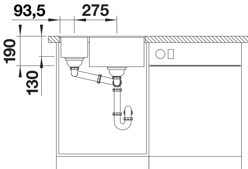
Vooraanzicht
