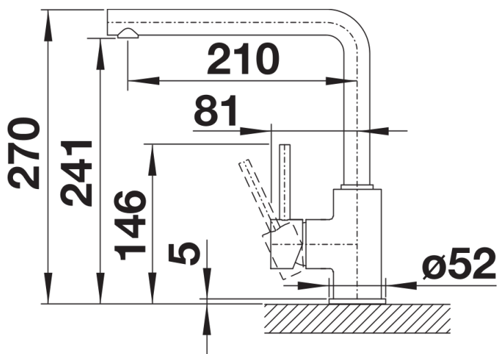
Zijaanzicht
