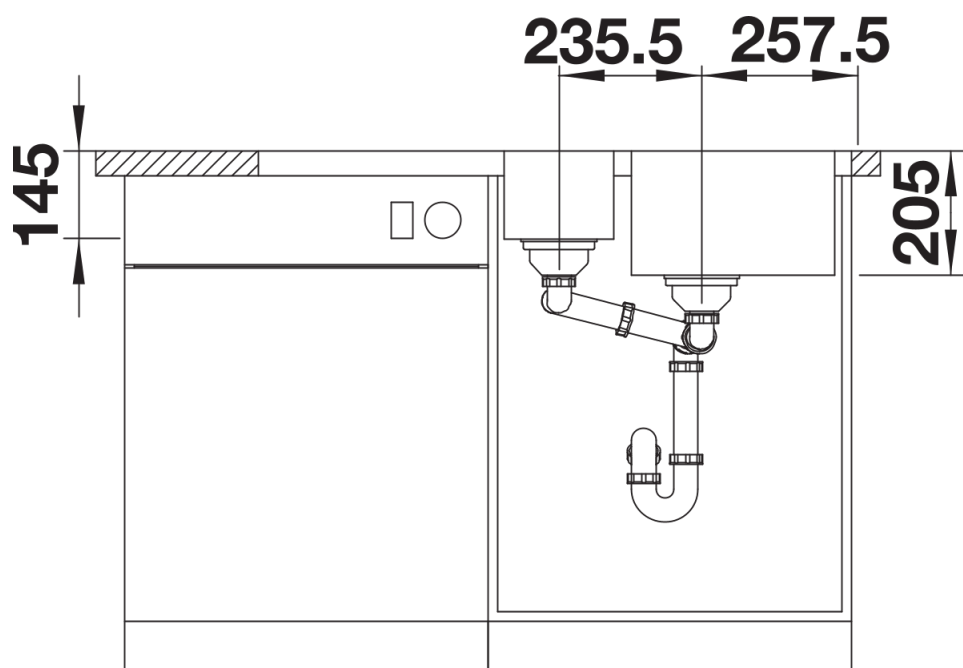
Vooraanzicht
